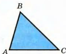
Трикутник ABC
